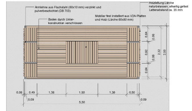
Grundriss
