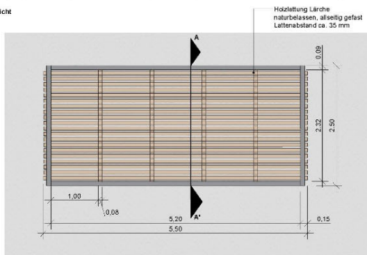
Draufsicht
