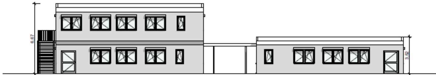
Ansicht NORD
